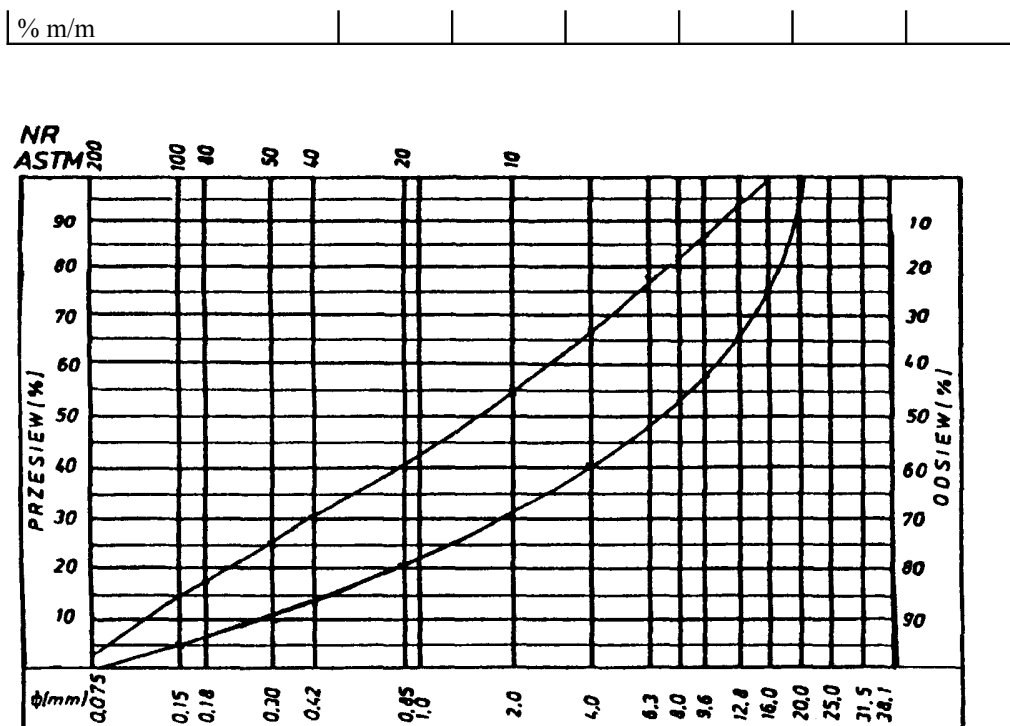
Rys. 8. Krzywe graniczne uziarnienia mieszanki mineralnej 0+20 mm do warstwy wiążącej, wyrównawczej i wzmacniającej z betonu asfaltowego dla KR 1-2
