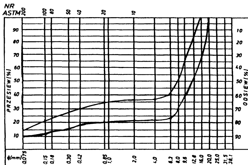
Rys. 5. Krzywe graniczne uziarnienia mieszanki mineralnej 0+20 mm o nieciągłym uziarnieniu do warstwy ścierniej z betonu asfaltowego dla KR 3-6
