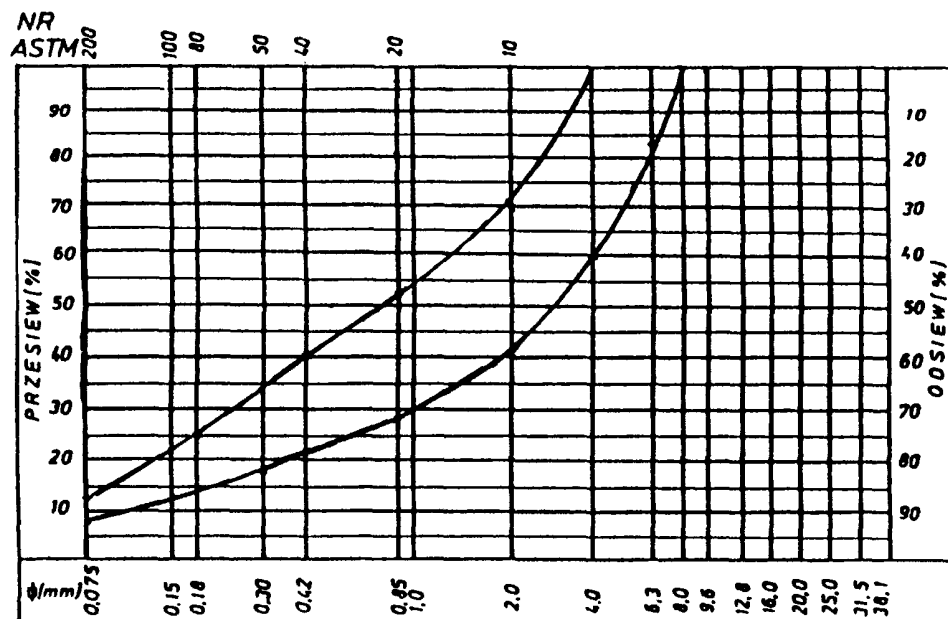
Rys. 3. Krzywe graniczne uziarnienia mieszanki mineralnej 0+8, 0+6,3 mm do warstwy ściernalnej z betonu asfaltowego dla KR 1-2
