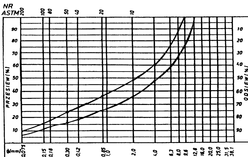
Rys. 6. Krzywe graniczne uziarnienia mieszanki mineralnej 0+16 mm do warstwy ścierniej z betonu asfaltowego dla KR 3-6
